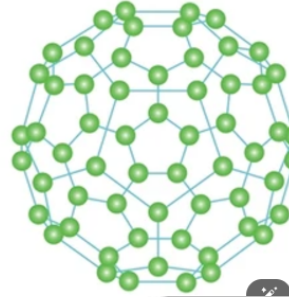
Fullerene
